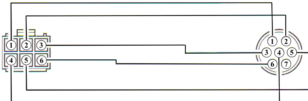
Hopkoppling av kontrollkabel (samma nummer på vardera kontakten används)
