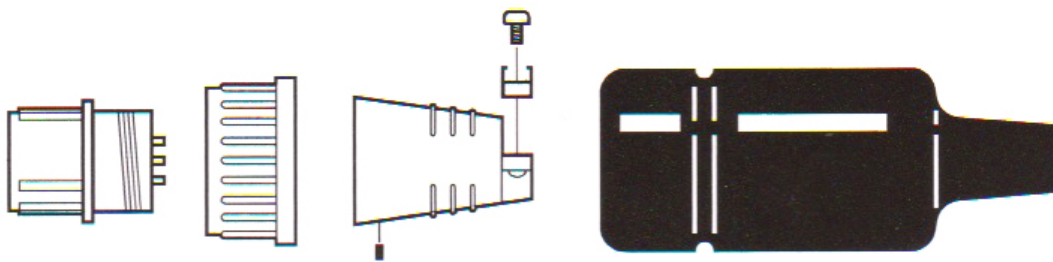
Montering av 7-polig rund Motorkontakt
