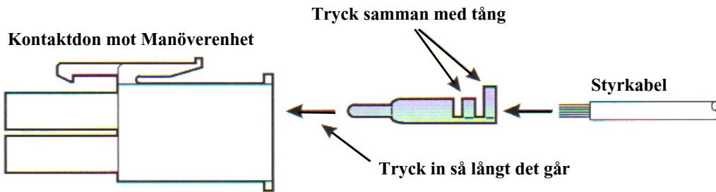
Montering av 6-polig rektangulär kontakt med stift
